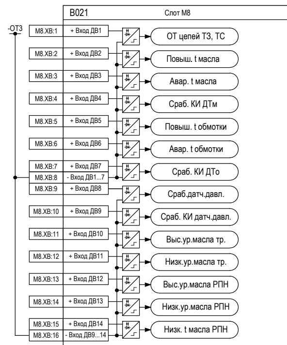
Рисунок Е.3 – Подключение дискретных входов и выходов к внутренним сигналам алгоритмов для плат в слотах М6-М8
