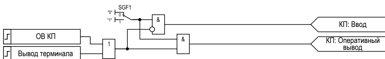
Рисунок 2.22 – Функциональная схема управления режимами работы «КП»
